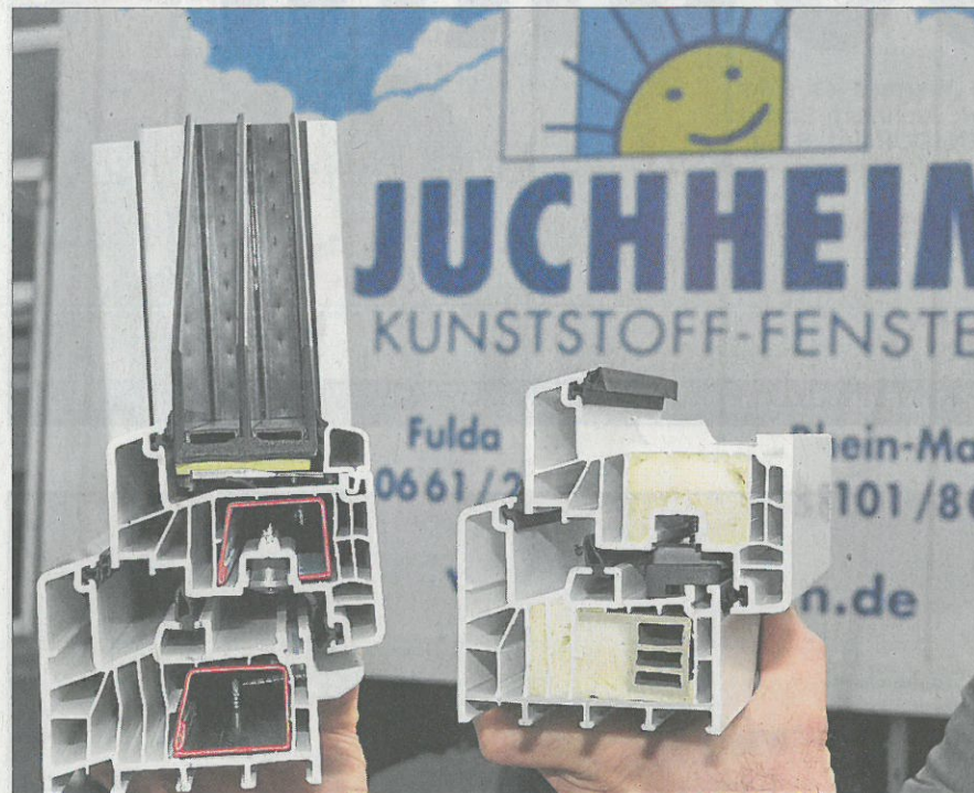
Bei dem neuen Fenstermodell Astro Therm Star ist das Profil mit Schaumstoff gefüllt. Die Dämmwerte sind so extrem hoch. Fotos: Volker Nies
